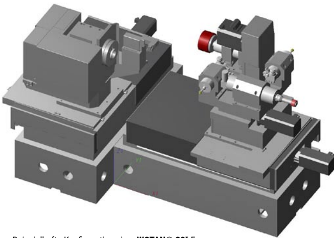
Beispielhafte Konfiguration einer WOTAN® S3I-F
