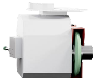
Außenschleifscheibe um 360° drehbar
