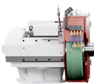
Außenschleifscheibe feststehend
